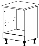
A/60/T-ALSÓ TŰZHELY TARTÓS 85 X 60 X 60
